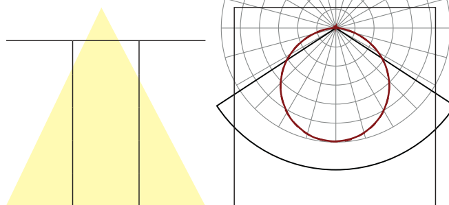
Lichtverteilungskurve
